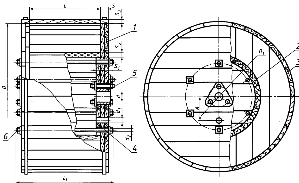
1 — щека; 2 — шейка; 3 — обшивка; 4 — круг шейки; 5 — втулка; 6 — шпилька
